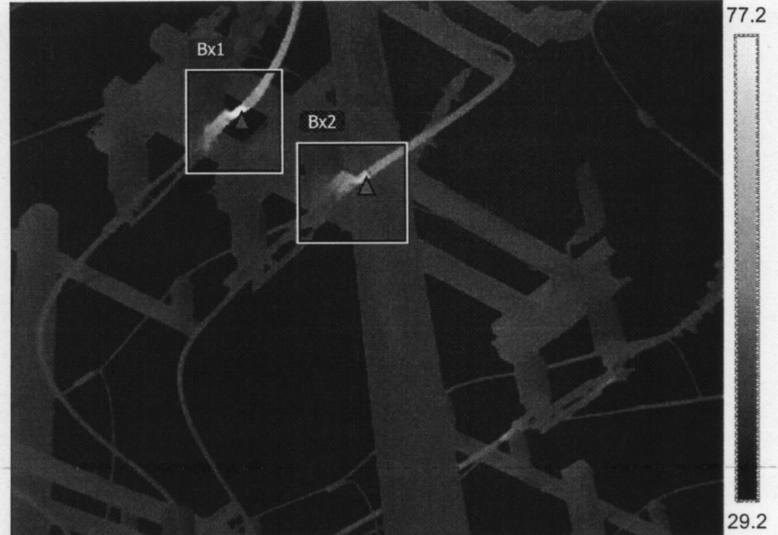
FLIR2716.jpg
