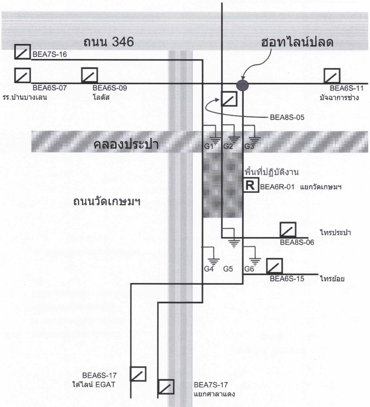
ผังดับไฟ 22 kV.แรงดัน วันที่ 4 กันยายน 2566 ทางเข้าวัดเกษมฯ
