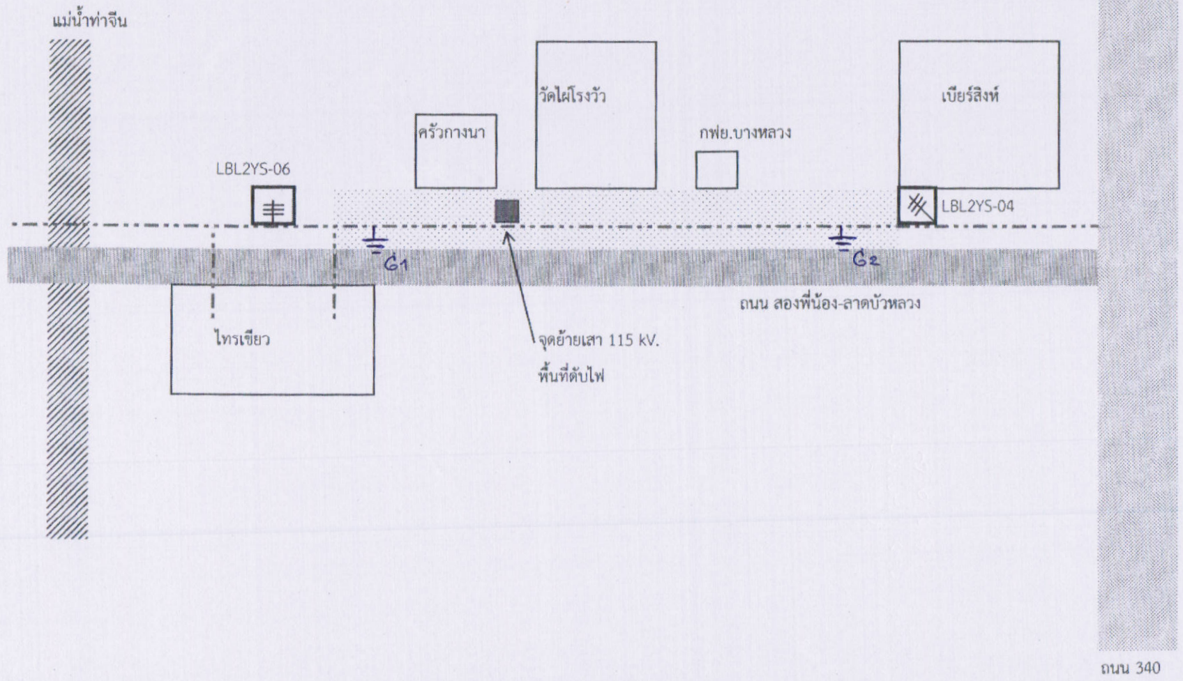
ผังงานดับไฟย้ายเสา 115 เควี บริเวณร้านครัววกางนา วัดไผ่โรงวัว
