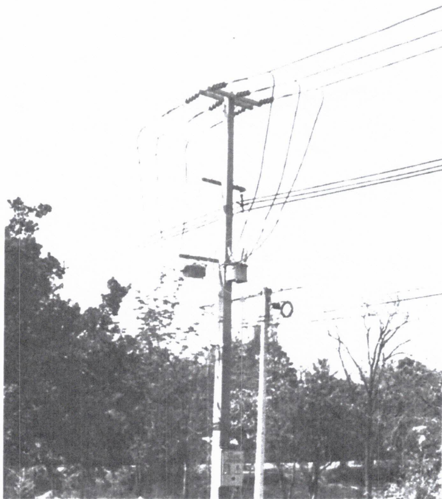
จุดปฏิบัติงานสับเปลี่ยน VT ของ SF๖ บ้านเสาชงษ์ รหัส BOP๐๑S-๐๒ โดยชุดหอไลน์
